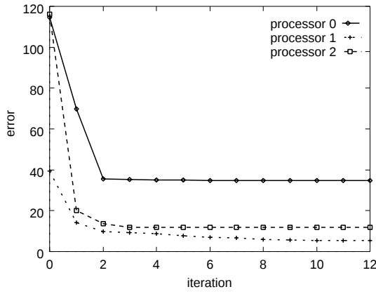
各プロセッサの平均 2 乗誤差の変化
