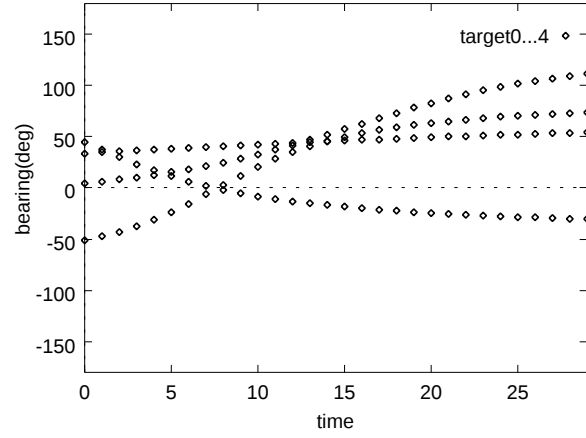
図 2: 多体軌跡推定におけるセンサの観測データの例
