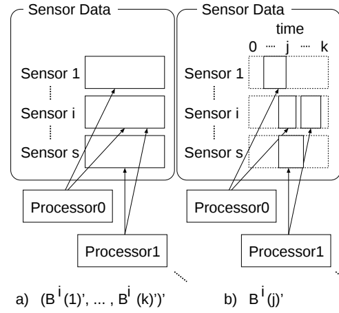
図 5: 観測データの選択における分割単位— a) 各センサのデータ (\beta^i(1)', \dots, \beta^i(k))' 単位での分割および b) 各センサ・各時刻のデータ \beta^i(j) 単位での分割
