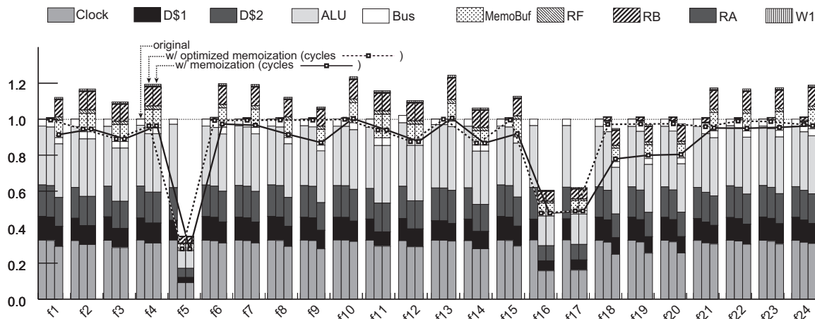
図 3 総消費エネルギー比 (GENEsYs)
