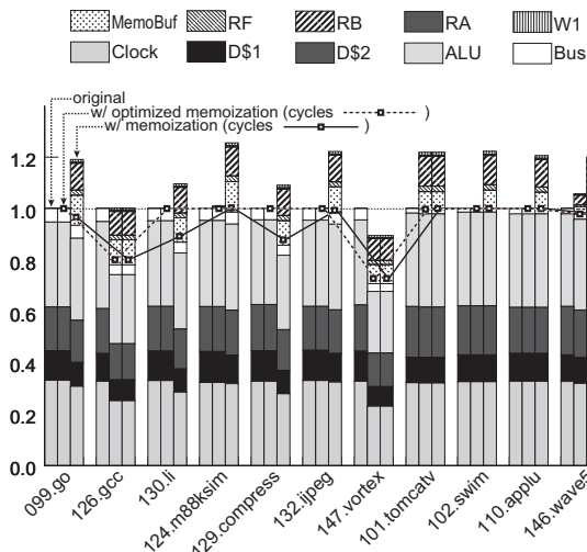
図 2 総消費エネルギー比 (SPEC CPU95)
